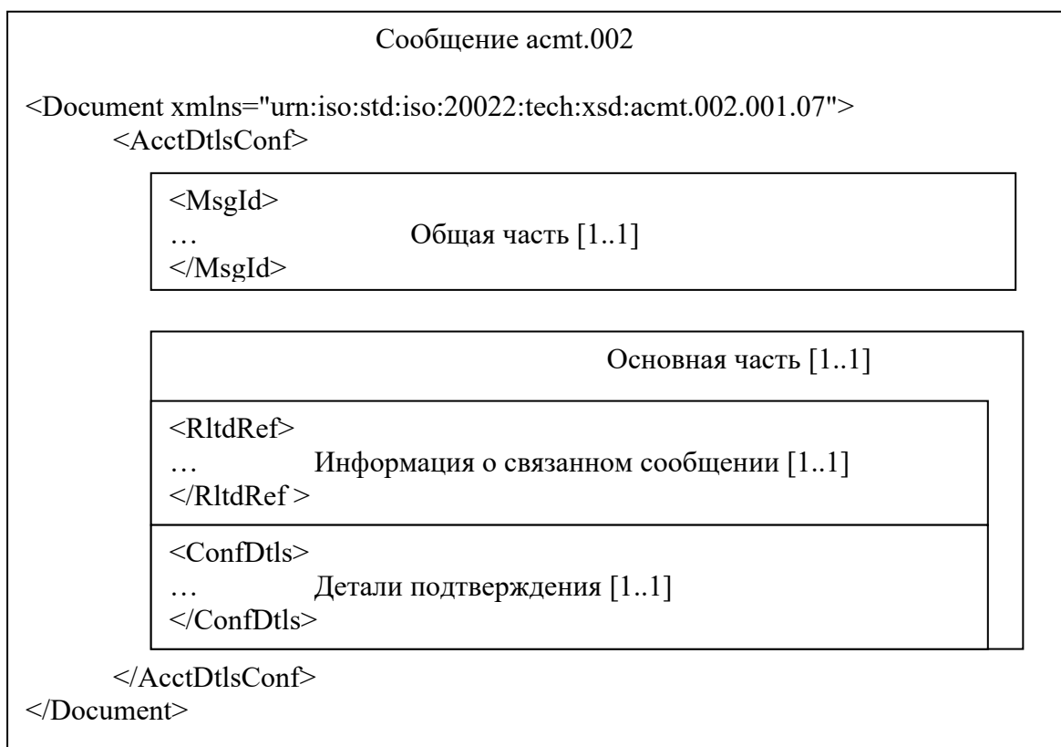
Рисунок 1 – Структура сообщения acmt.002
