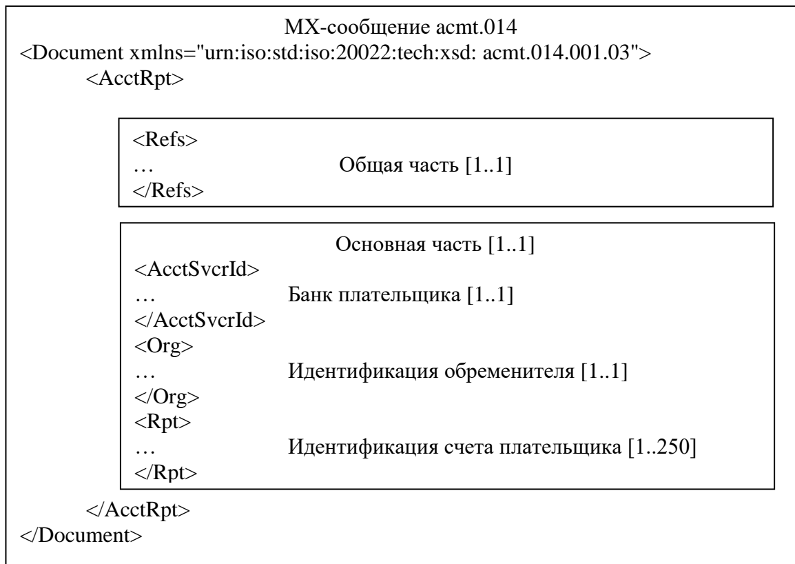
Рисунок 1 – Структура МХ-сообщения acmt.014
