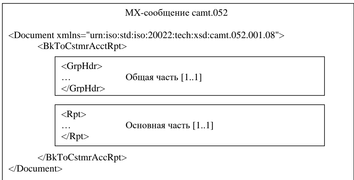
Рисунок 1 – Структура МХ-сообщения camt.052
