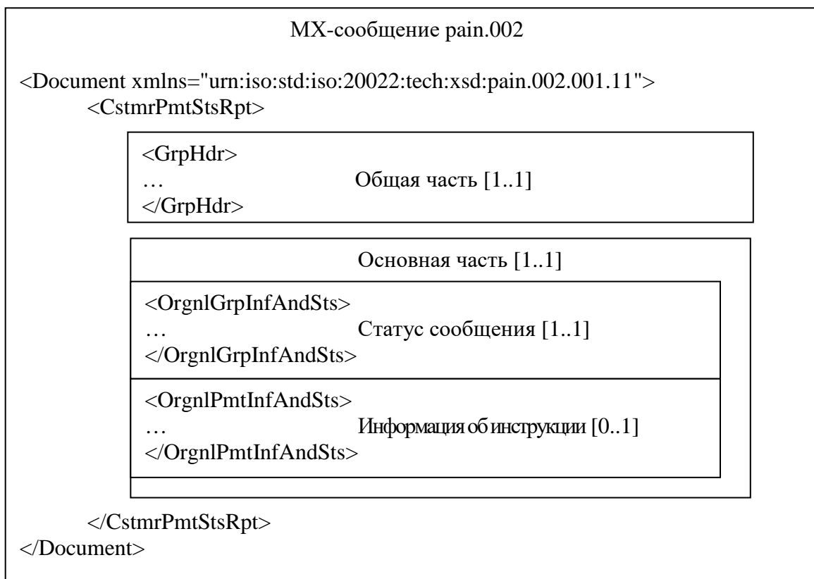
Рисунок 1 – Структура МХ-сообщения pain.002
