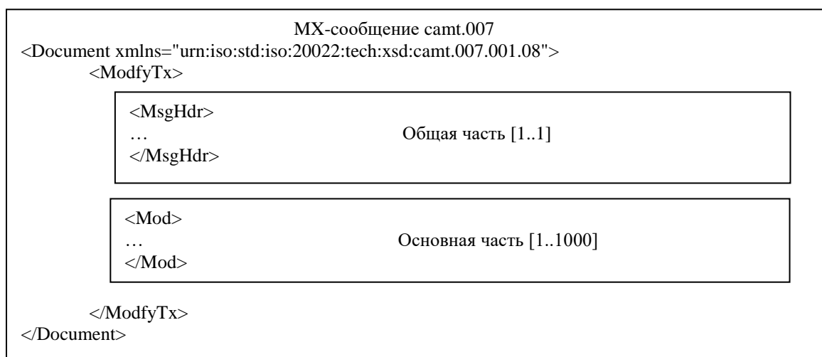
Рисунок 1 – Структура МХ-сообщения camt.007
