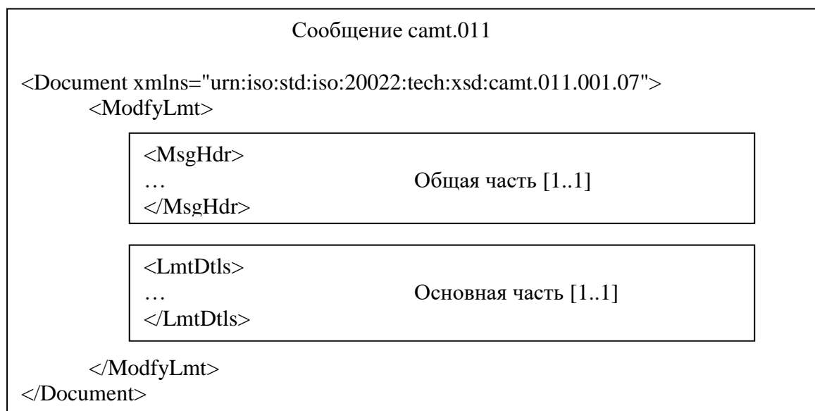
Рисунок 1 – Структура сообщения camt.011
