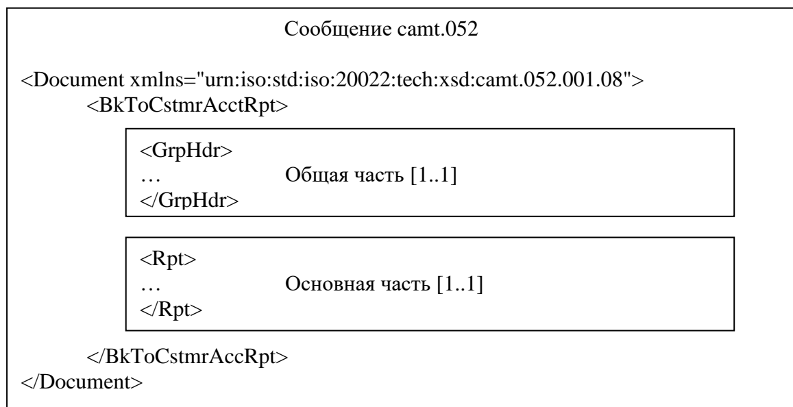
Рисунок 1 – Структура сообщения camt.052
