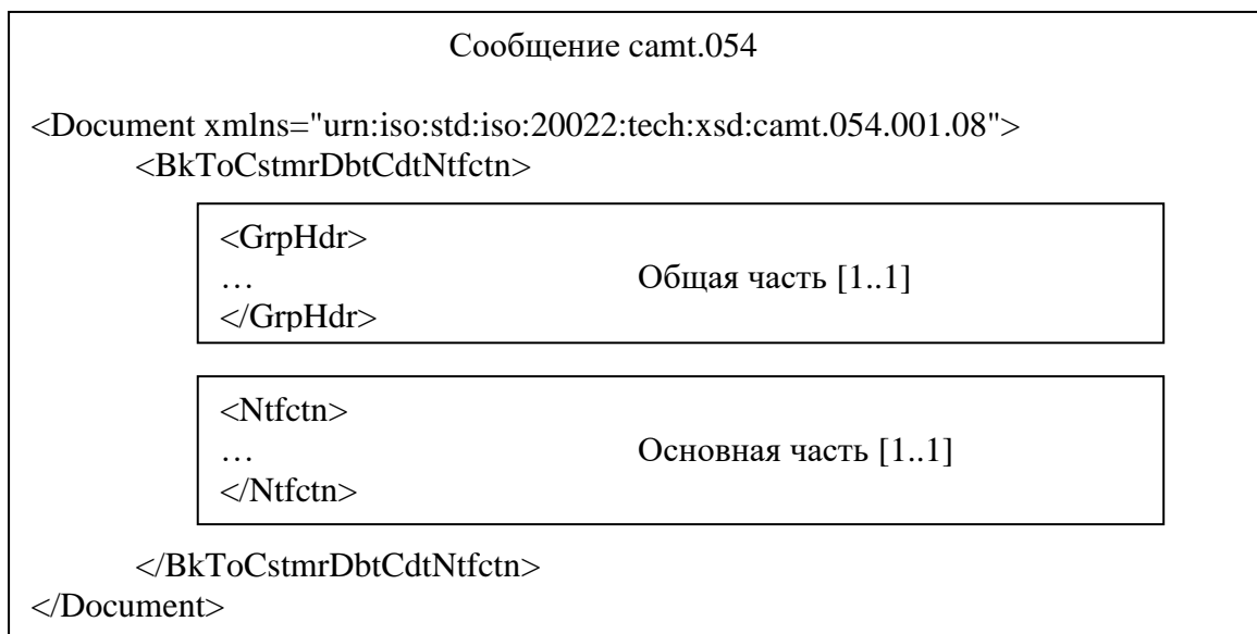
Рисунок 1 – Структура сообщения camt.054
