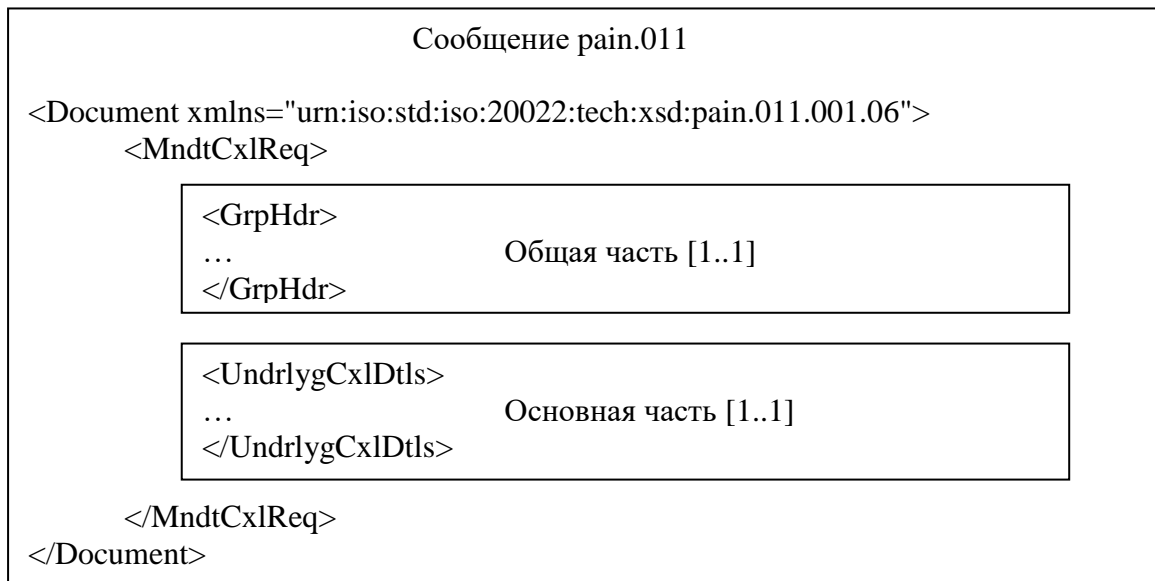
Рисунок 2 – Структура сообщения pain.011
