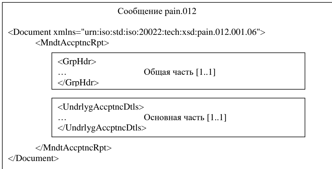
Рисунок 3 – Структура сообщения pain.012
