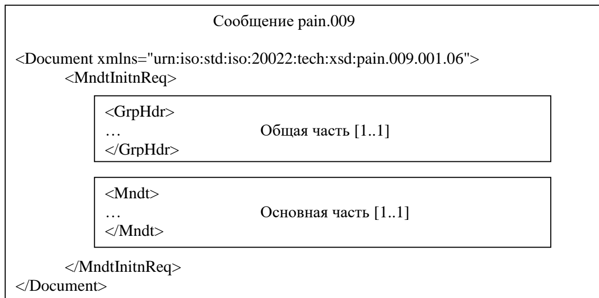
Рисунок 1 – Структура сообщения pain.009
