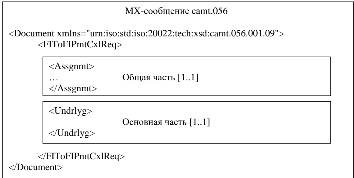
Рисунок 1 – Структура МХ-сообщения camt.056
